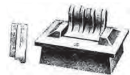
IM008 Self Action Gate Stop in Grey Iron H113 x W113 x D3mm Cl:3.0kg H187 x W156 x D7mm Cl:7.0kg H245 x W181 x D13mm Cl:13.0kg H300 x W213 x D20mm Cl:20.0kg H375 x W386 x D34mm Cl:34.0kg 363 x W313 x D69mm Cl:69.0kg
