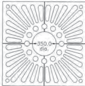
G008 1220 x 1220 x 350 I/D x 25mm Thick Cl:86kg
