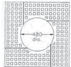
G003 925 x 925 x 480 I/D x 25mm Thick Cl:84kg
