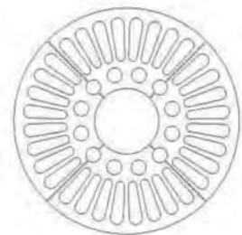
G005 1220 O/D x 350 I/D x 20mm Thick Cl:88kg
