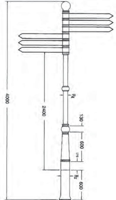
A263 Post: Cl:117kg Finger: Cl:13kg
