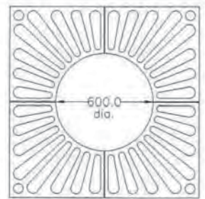
G013 1170 x 1170 x 600 I/D x 25mm Thick Cl:284kg
