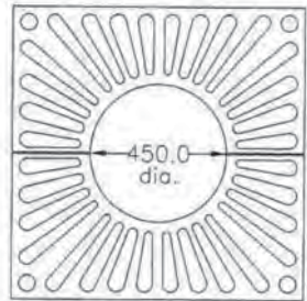
G010B 968 x 968 x 450 I/D x 25mm Thick Cl:84kg
