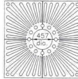
G011 1768 x 1768 x 457 I/D x 25mm Thick Cl:284kg
