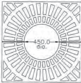
G007A 1014 x 1014 x 450 I/D x 25mm Thick Cl:86kg
